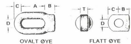
ØYEBOLTER
